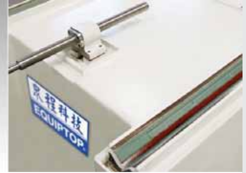
Ansicht der geschabten V-Flachführungen in der X-Achse.
