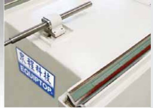
Ansicht der geschabten V-Flachführungen in der X-Achse.
